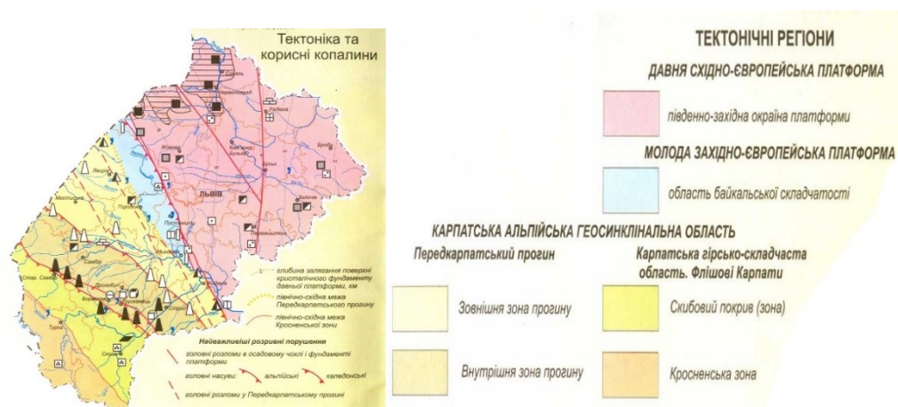
Рис. 2.6. Тектонічні особливості Львівської області 15
